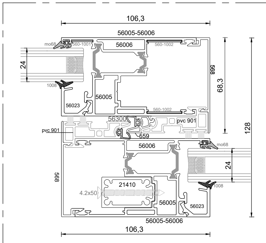
lift & slide-300kg
