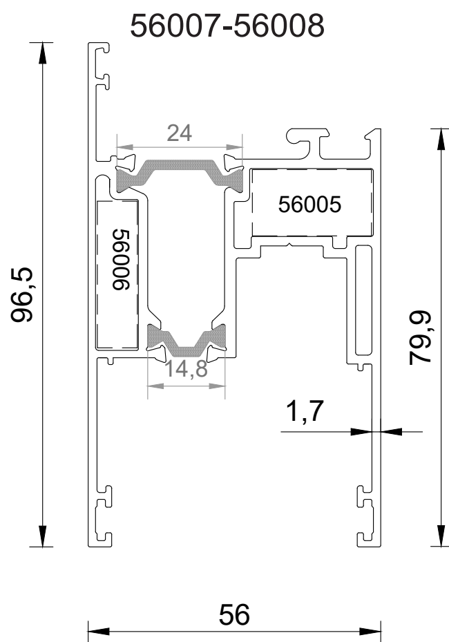
200 kg-big sash profil
